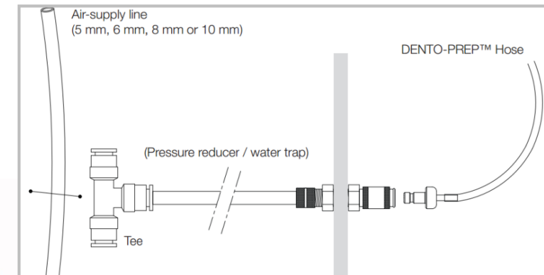
Installation Kit til slange-diameter 5mm Varenr. 1925
